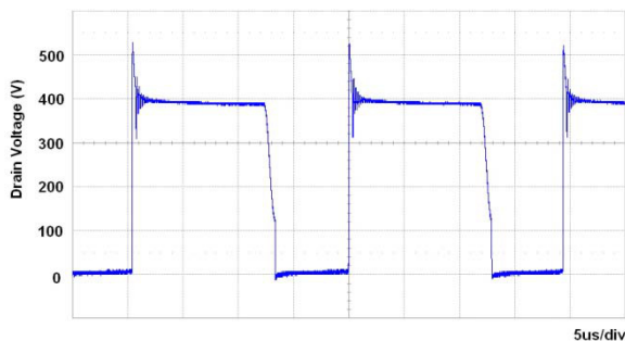
图 17. 第一谷底开关
