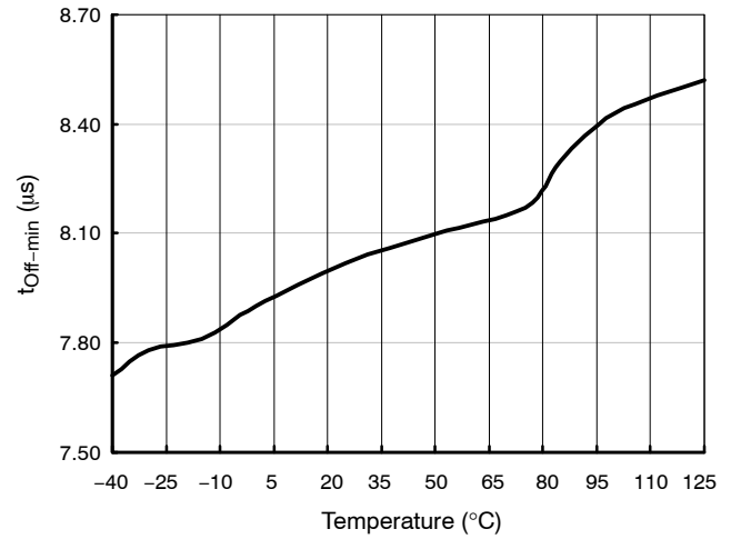
图 13. 最小关断时间 (V FB > V N )
