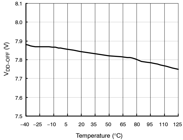
图 4. 导通阈值电压
