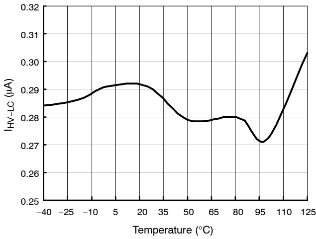
图 10. 启动后漏电流
