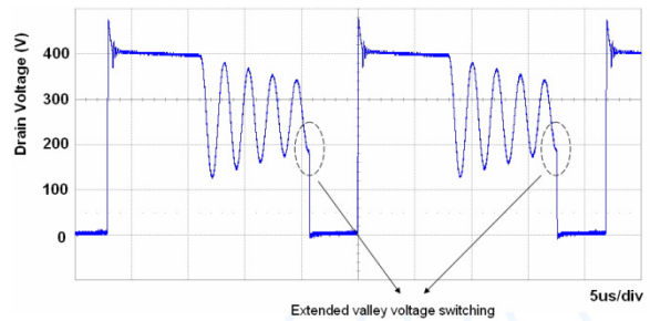
图 19. 扩展波谷电压检测模式下 QR 工作波形
