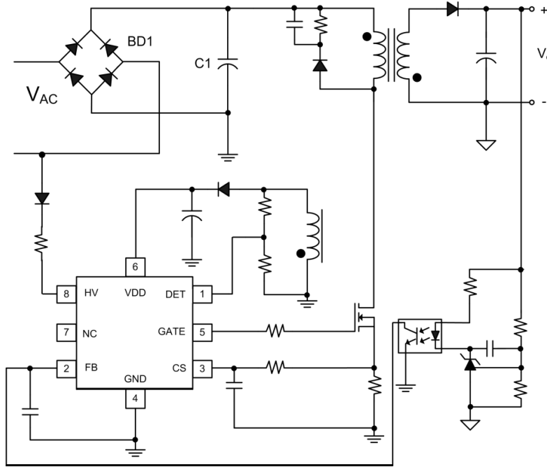
图 1. 典型应用
