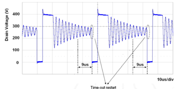
图 20. 内部 t_{TIME-OUT} 在未能检测波谷电压后会启动新周期 (FAN6300H 版本中为 5 \mu s 延迟)
