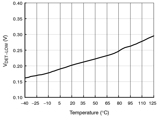
图 11. 箝位电压下限
