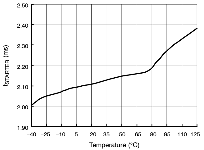
图 15. 启动计时器 (V FB < V G )
