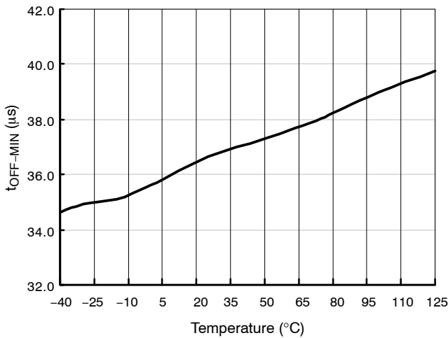
图 14. 最小关断时间 (V FB = V G )
