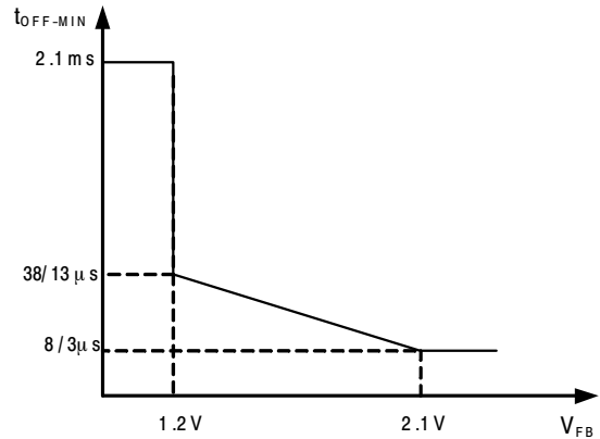
图 18. V_{FB} 与 t_{OFF-MIN} 曲线的关系
