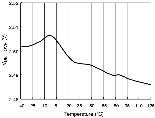
图 12. 比较器参考电压
