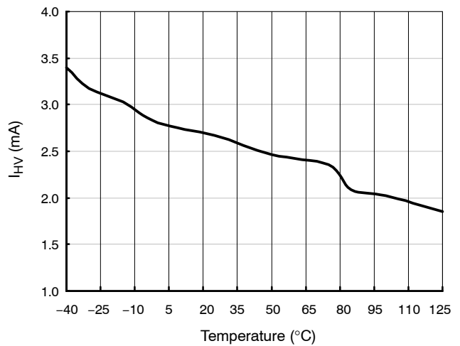
图 9. 从引脚 HV 可提供电流
