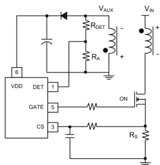
图 21. 通过 DET 引脚补偿高/低压电压的恒功率限值
