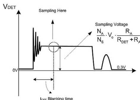
图 22. 栅极关断后， 4 \mu s (FAN6300H 版本为 1.5 \mu s ) 的消隐时间过后采样得到的电压
