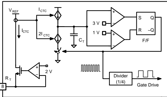
图 17. 电流控制的振荡器
