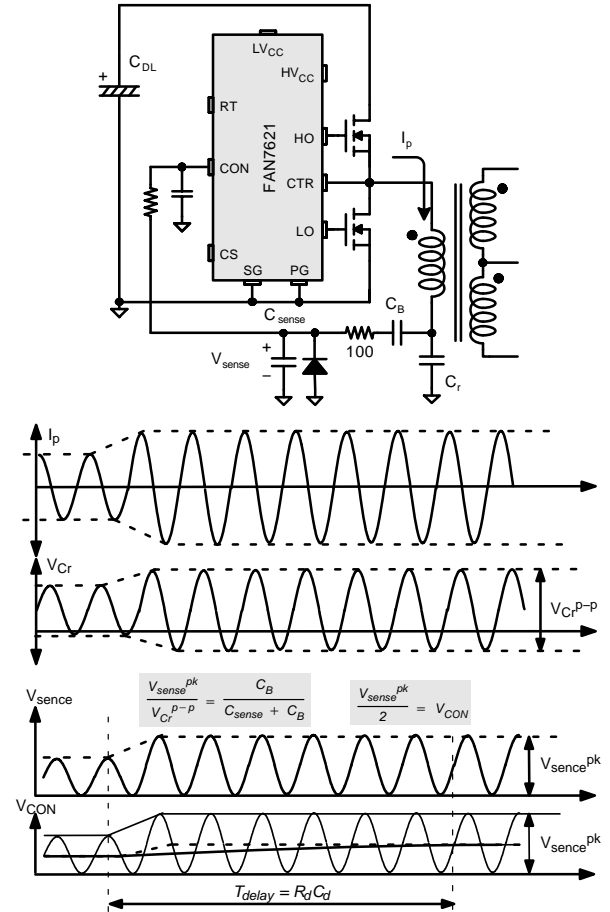
图 27. 使用谐振电容电压的电流感测
