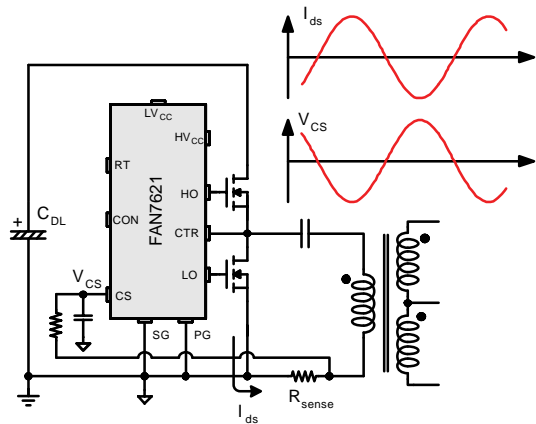
图 26. 全波检测
