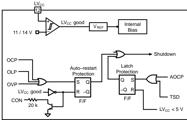
图 24. 保护框图
