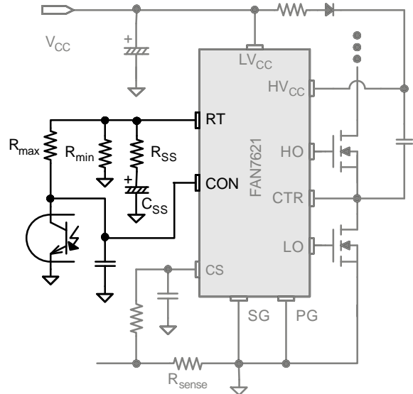
图 19. 频率控制电路
