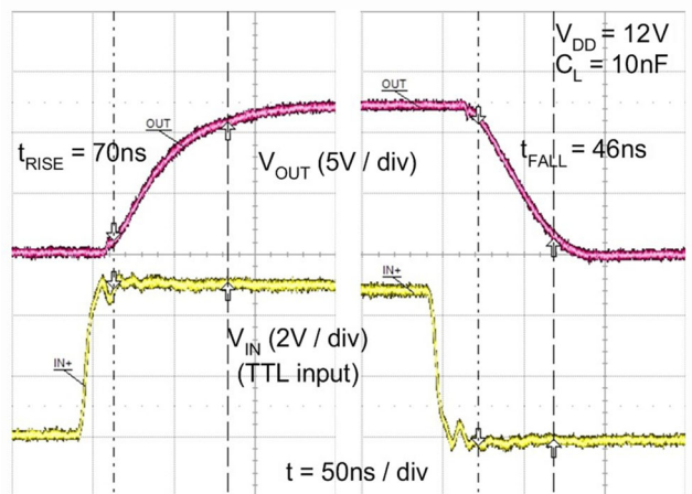
图 32. 上升/下降波形, 10 nF 负载
