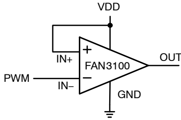
图 42. 使能的双输入驱动器，反相配置
