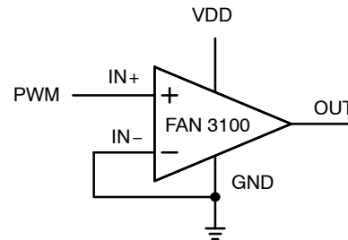
图 41. 使能的双输入驱动器，同相配置
