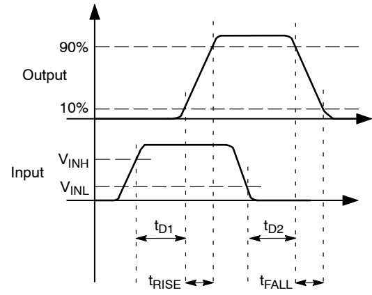
图 3. 同相
