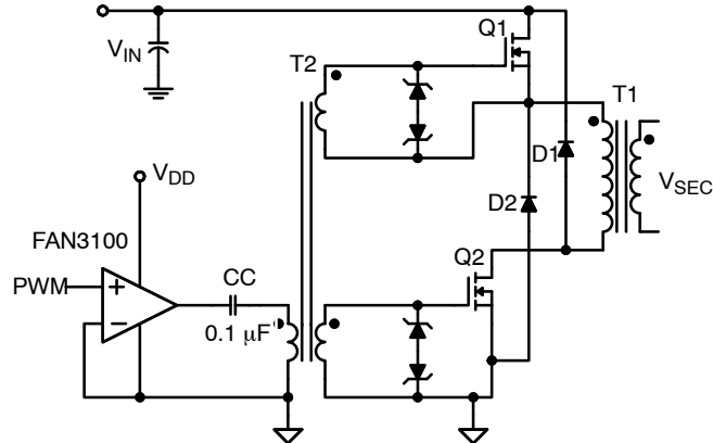
图 46. 双晶体管正向转换器栅极变压器的驱动器
