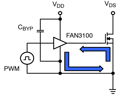
图 40. MOSFET 关断时的电流通路
