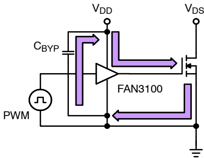
图 39. MOSFET 导通时的电流路径
