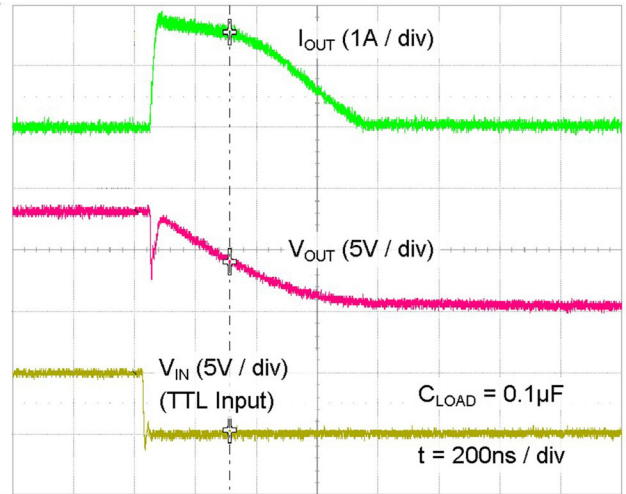
图 36. V_{DD} = 8\text{ V} 时的准静态灌电流波形
