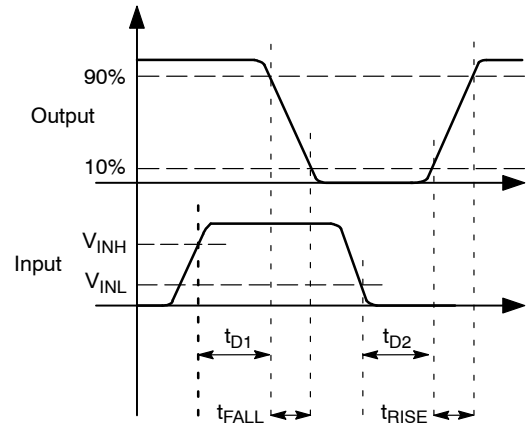
图 4. 反相
