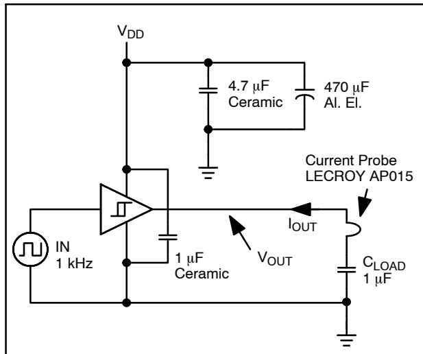
图 37. 准静态 I_{OUT}/V_{OUT} 测试电路
