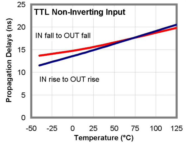
图 25. 传播延迟与温度的关系
