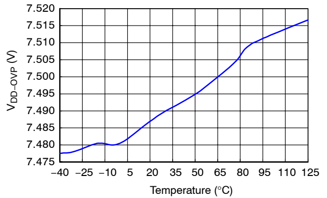
图 9. V_{VREF} 与温度的关系
