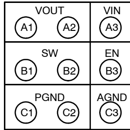
图 3. 俯视图
