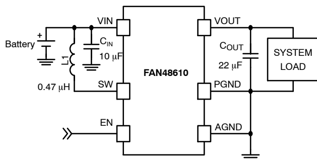
图 1. 典型应用
