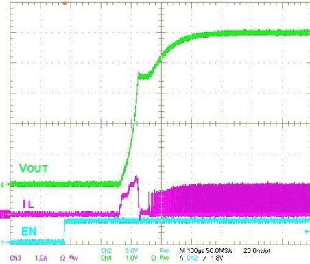
图 14. 启动，50 \Omega 负载
