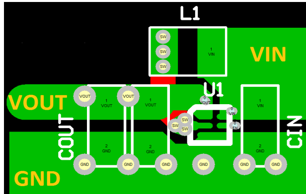
图 22. 推荐布局
