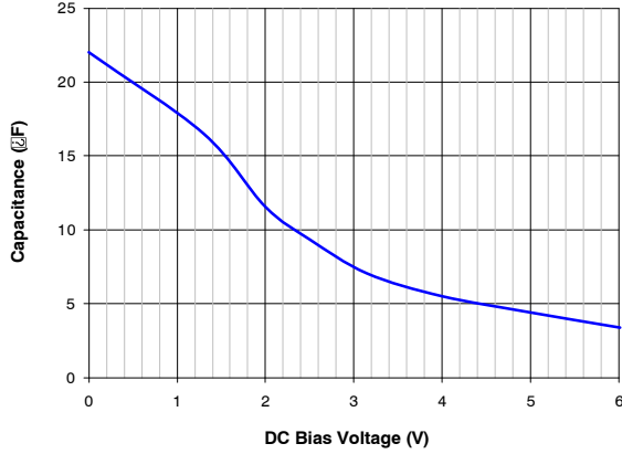
图 21. 22 μF、0603、X5R、6.3 V额定电容的 C EFF (TDK C1608X5R0J226M)
