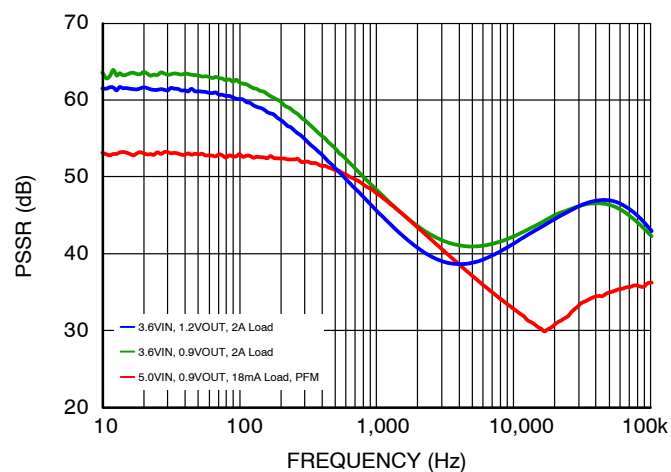
图 22. PSRR vs. 频率
