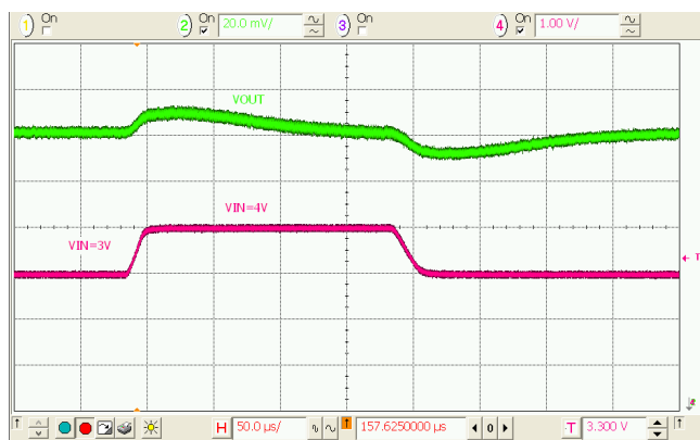
图 24. 线路瞬态，3-4 V_{IN} ，1.2 V_{OUT} ，10 \mu\text{s} 边沿，1 A 负载
