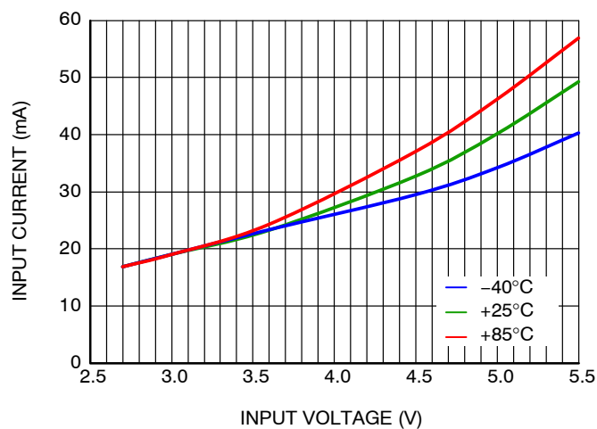
图 20. 静态电流与输入电压和温度的关系，FPFM
