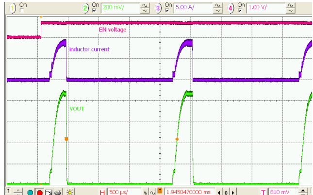
图 33. 启动持续到负载出现故障， V_{OUT} = 0.9\text{ V}
