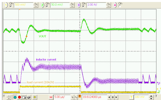
图 26. 负载瞬态， 3.6\text{ V}_{IN} ， 1.2\text{ V}_{OUT} ， 0.3\text{--}3\text{ A} ， 100\text{ ns} 边沿
