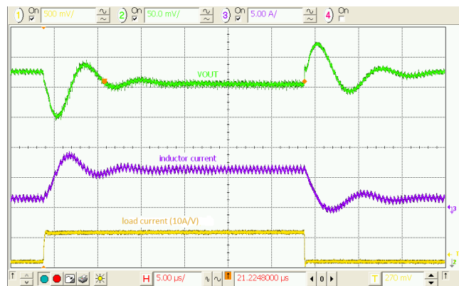
图 28. 负载瞬态， 3.6\text{ V}_{IN} ， 1.2\text{ V}_{OUT} ， 1.5\text{--}6\text{ A} ， 100\text{ ns} 边沿， C_{OUT} = 4 \times 22\text{ }\mu\text{F}
