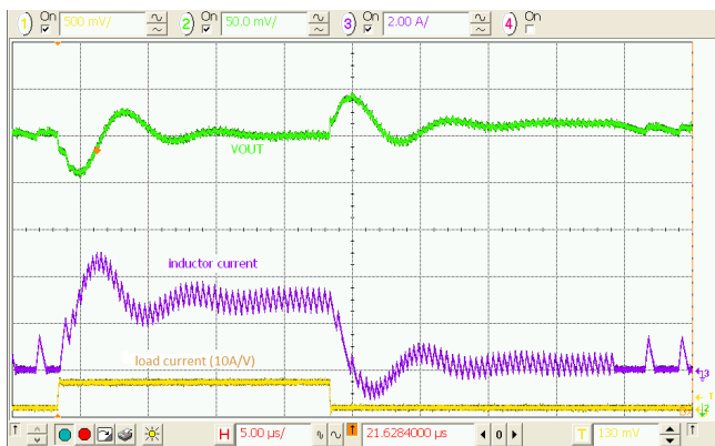
图 27. 负载瞬态， 3.6\text{ V}_{IN} ， 1.2\text{ V}_{OUT} ， 0.3\text{--}3\text{ A} ， 100\text{ ns} 边沿， C_{OUT} = 4 \times 22\text{ }\mu\text{F}
