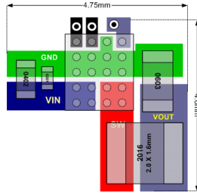
图 2. 减小尺寸的布局
