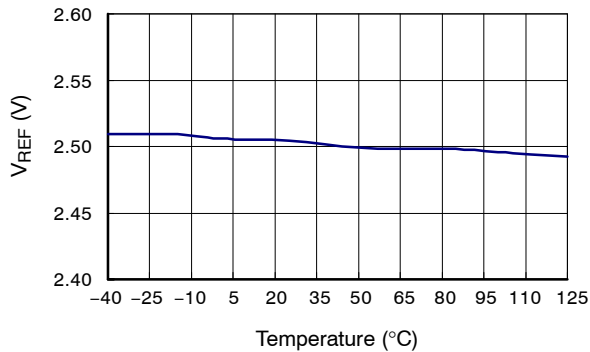
图 10. PFC 输出反馈参考电
