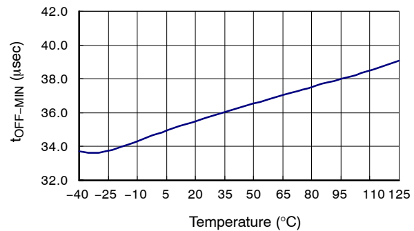
图 19. VFB 的 PWM 最小关断时间 = VG
