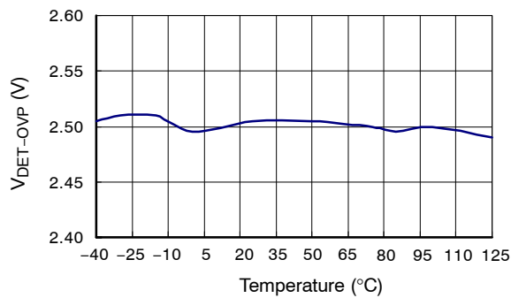
图 21. DET 引脚过压保护参考电压
