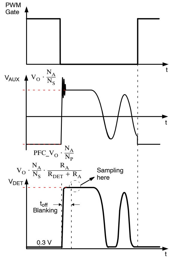
图 43. 输出过压检测工作波形
