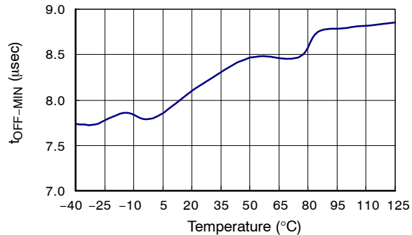
图 18. VFB 的 PWM 最小关断时间 > VN
