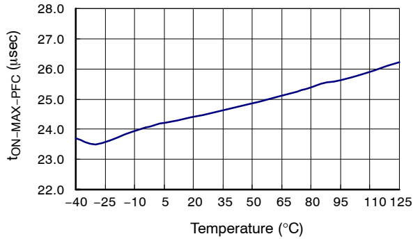
图 12. PFC 最大导通时间
