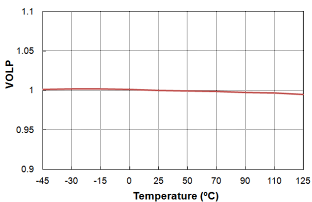
图 31. VOLP 与温度的关系
