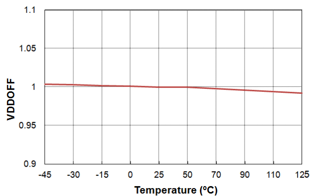
图 18. VDDOFF 与温度的关系
