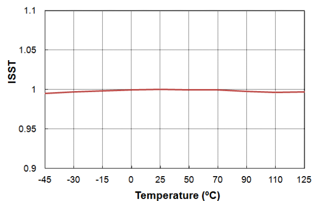
图 30. ISST 与温度的关系
