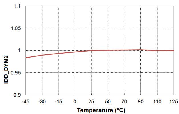
图 16. IDD_DYM2 与温度的关系
