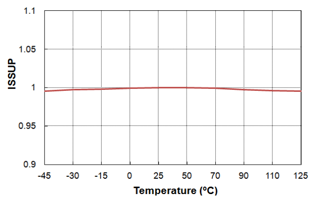
图 32. ISSUP 与温度的关系
