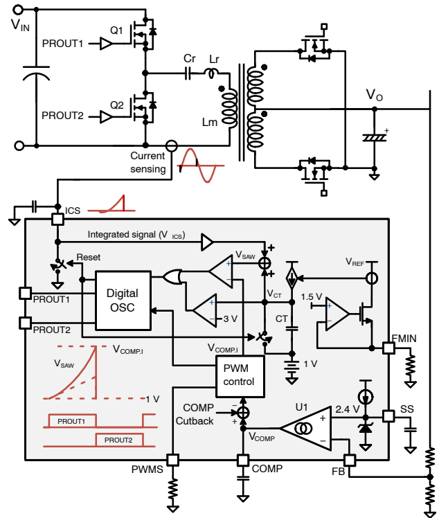
图 55. LLC 谐振转换器功率级的示意图
