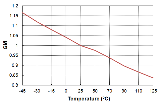
图 20. GM 与温度的关系
