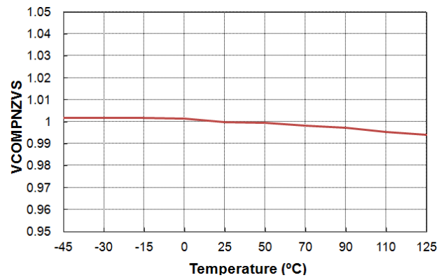
图 53. VCOMPNZVS 与温度的关系
