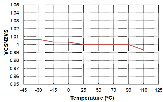
图 52. VCSNZVS 与温度的关
