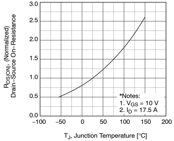
图 8. 导通电阻变化与温度的关系
