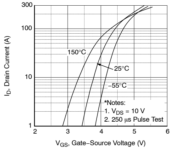
图 2. 传输特性
