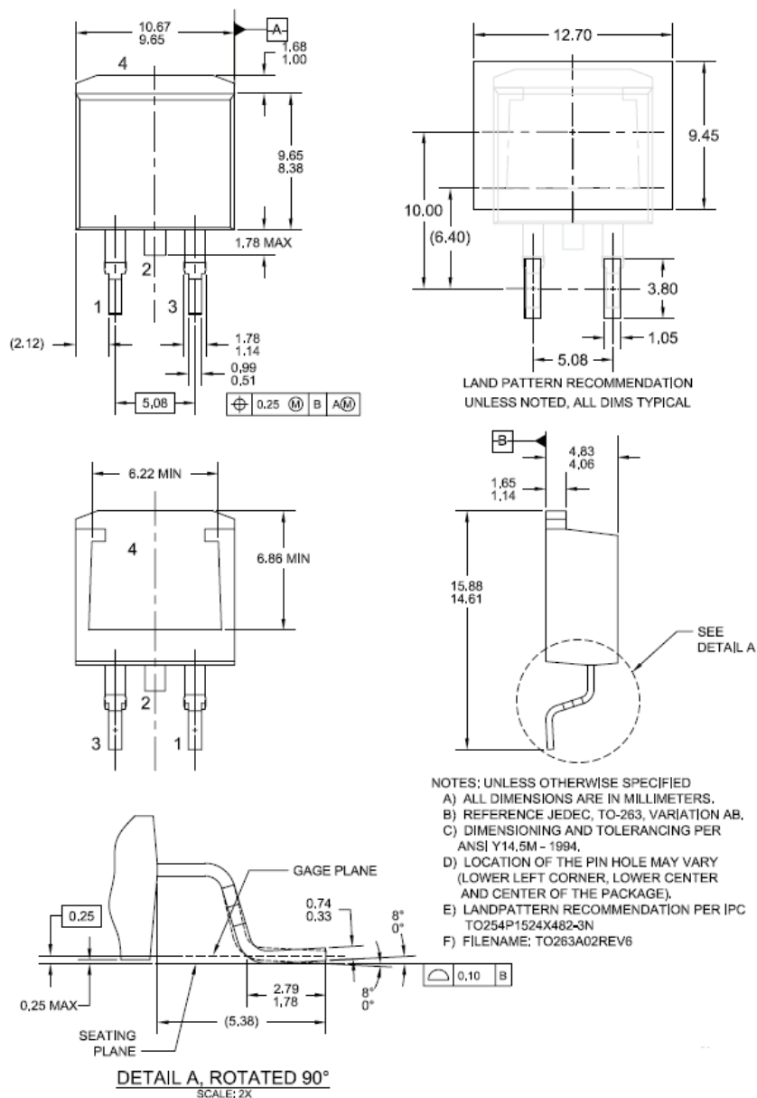
图 18. TO263 (D²PAK) 模塑 2 引脚表面贴装
