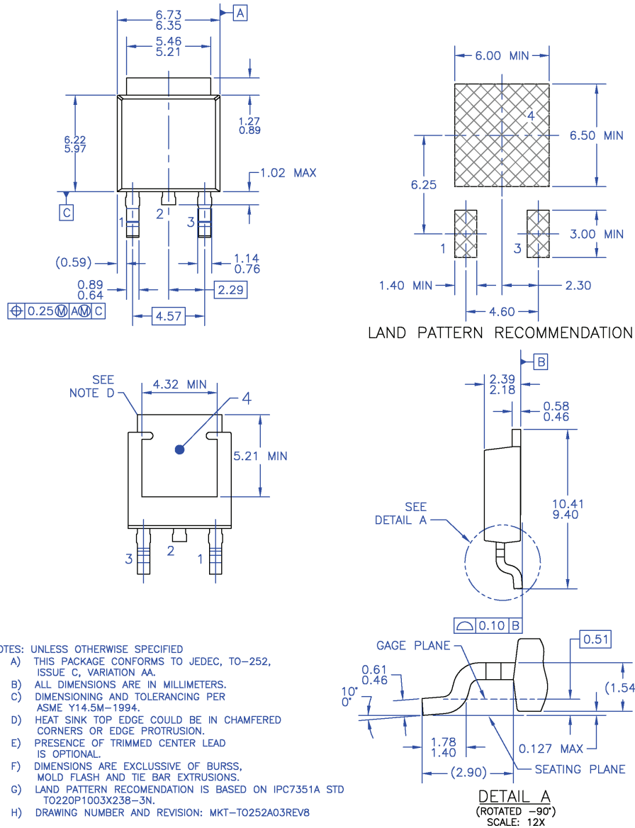
图 18. TO252 (D-PAK) 模塑 3 引线选项 AA&AB
