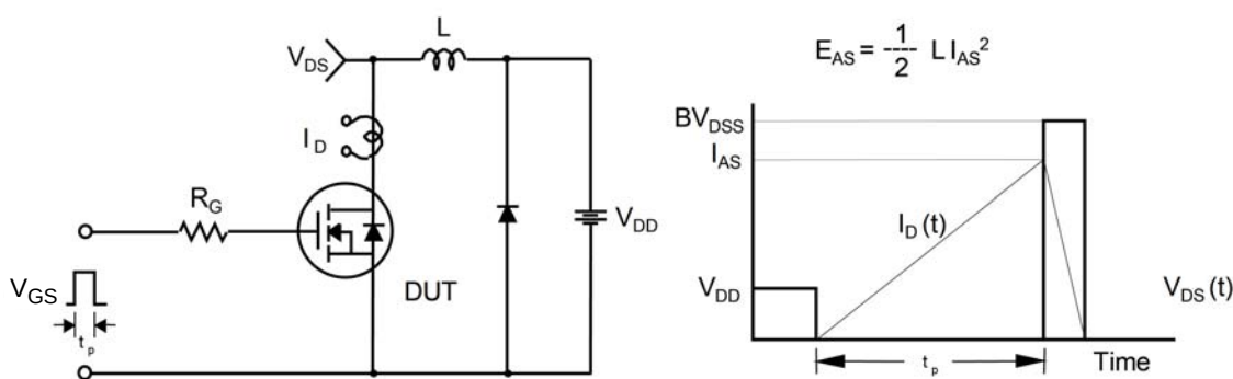
图 16. 非箝位电感开关测试电路与波形
