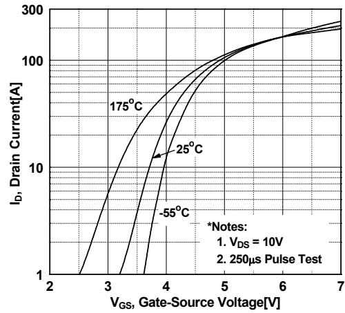
图 2. 传输特性
