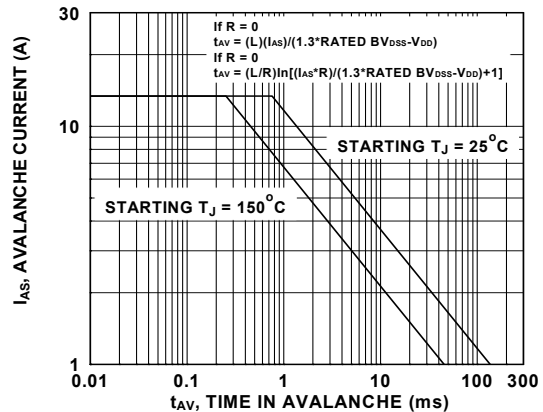
图 12. 非箝位电感开关能力
