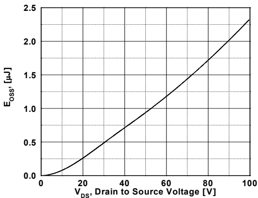
图 11. E_oss 和漏极 - 源极电压的关系
