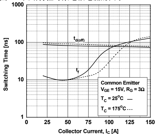
图 13. 关断特性与集电极电流的关系
