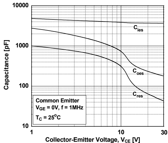
图 7. 电容特性
