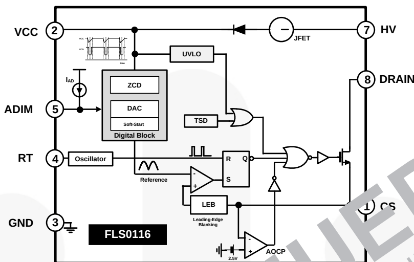
图2. 框图
