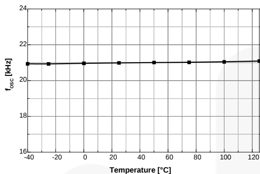
图19. f_{osc} 与温度的关系 ( R_T=87k\Omega )
