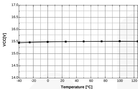
图13. V_{OV} 与温度的关系
