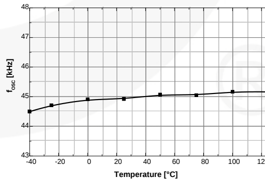
图18. f_{osc} 与温度的关系 (RT= 开路)
