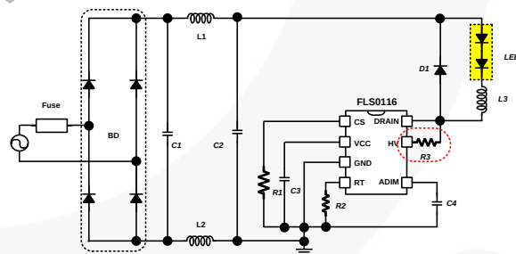
图6. 高压应用
