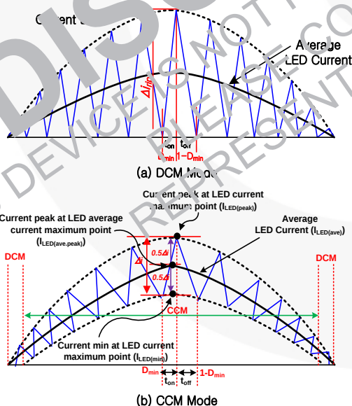
图8.DCM 和 CCM 运行
