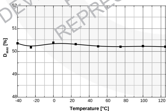
图23. D_{max} 与温度的关系
