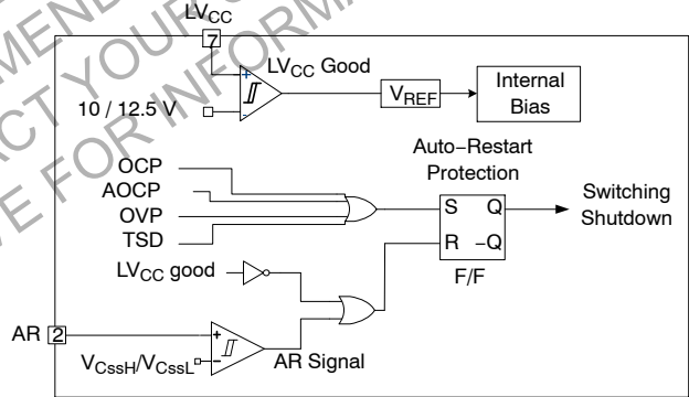
图 22. 保护框图
