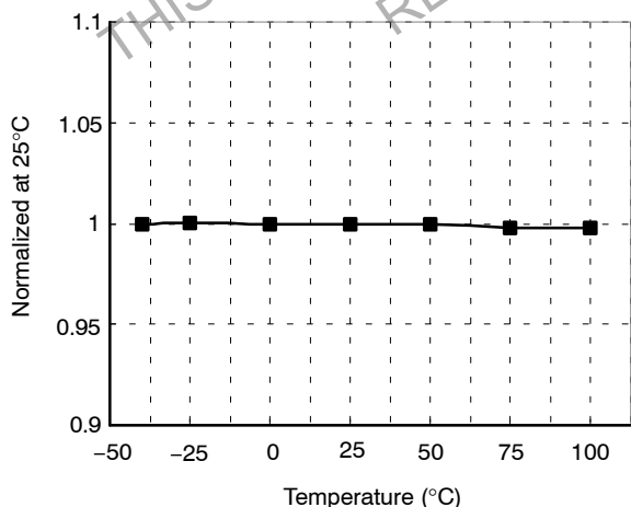
图 8. 低侧 V_{CC} (LV CC ) 开始与温度的关系
