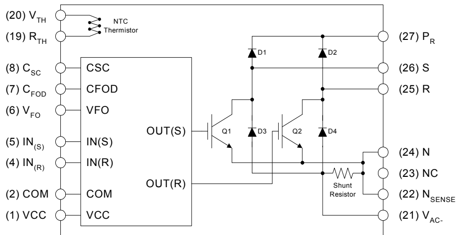
图 3. 内部框图
