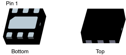
WDFN6 2x2, 0.65P CASE 511CY
