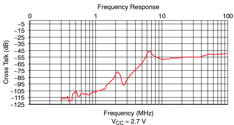
图 7. 串扰
