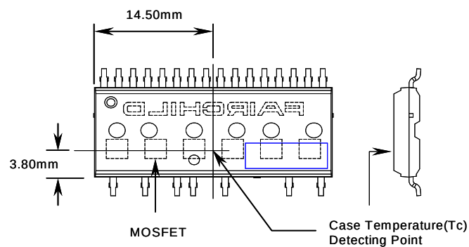
图 4. 壳体温度测量
