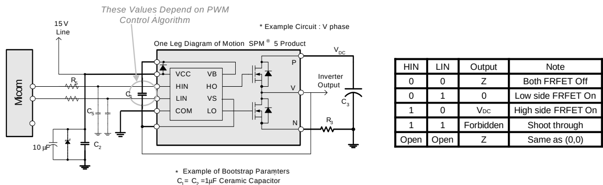
图 3. 推荐的 MCU 接口和自举电路及其参数
