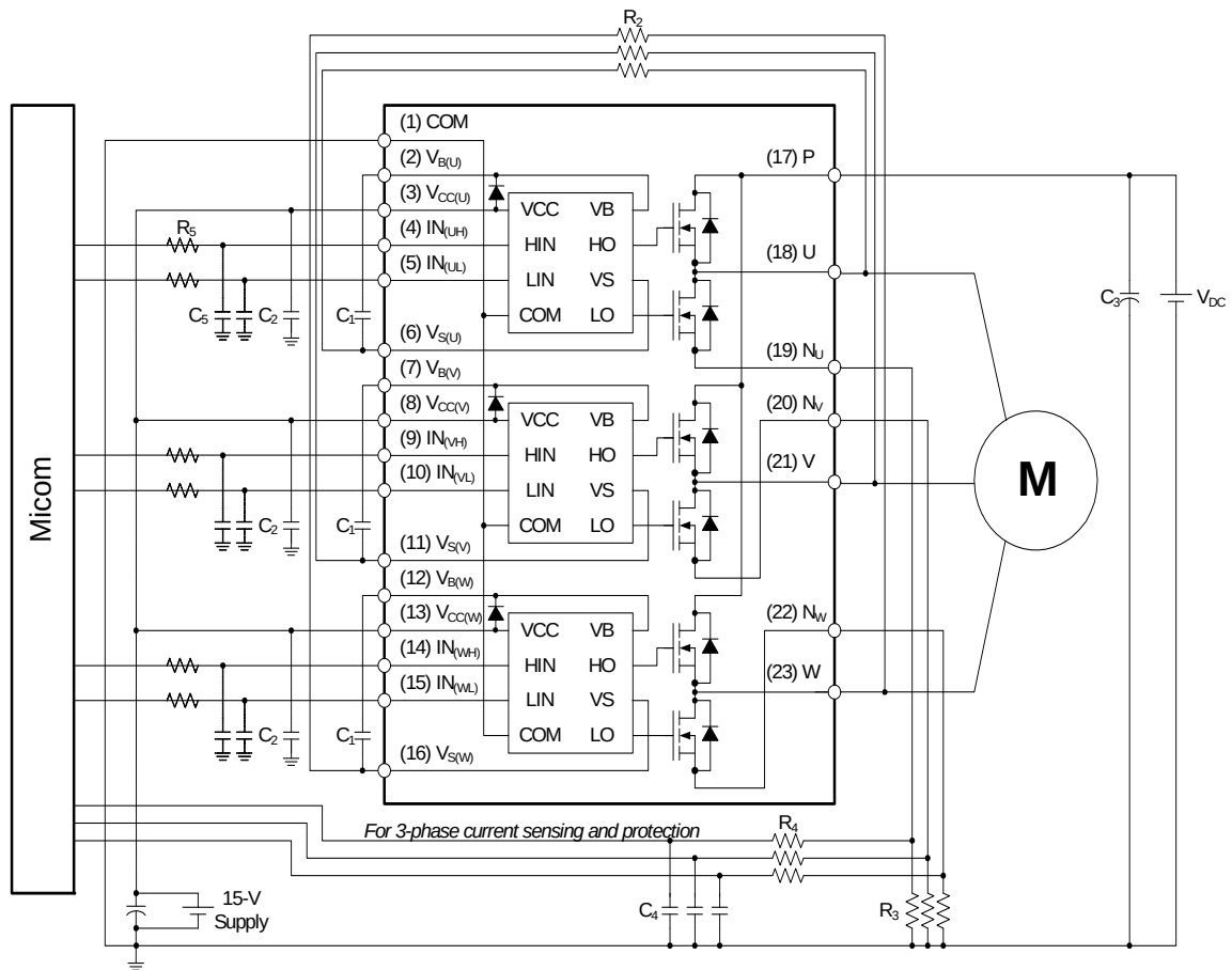
图 9. 应用电路实例
