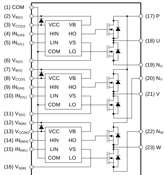
图 1. 引脚布局和内部框图（仰视图）
