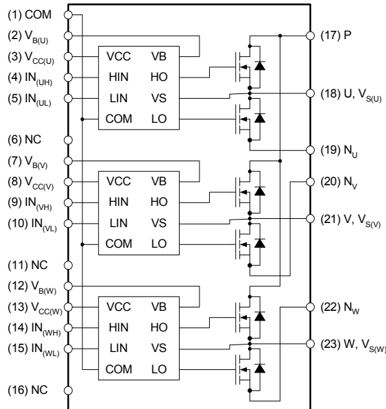
图 1. 引脚布局和内部框图（仰视图）
