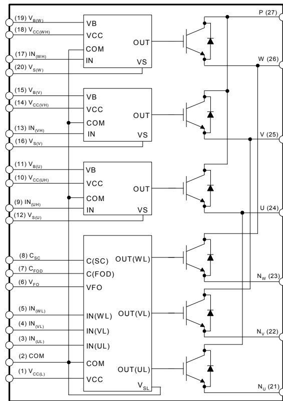
图 3. 内部框图
