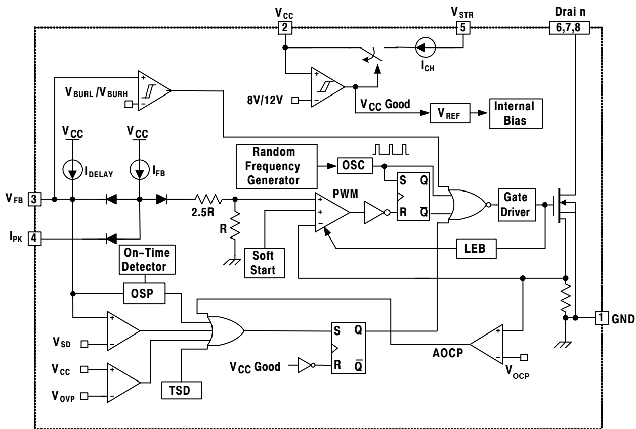
图 2. 内部框图
