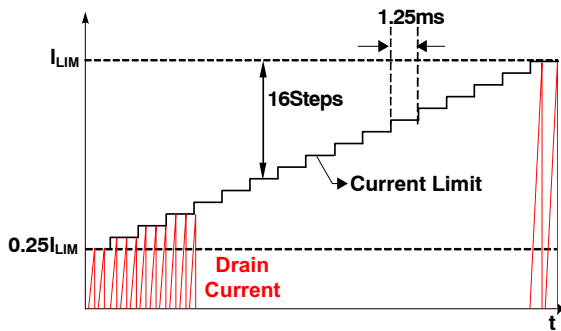
图 21. 内部软启动
