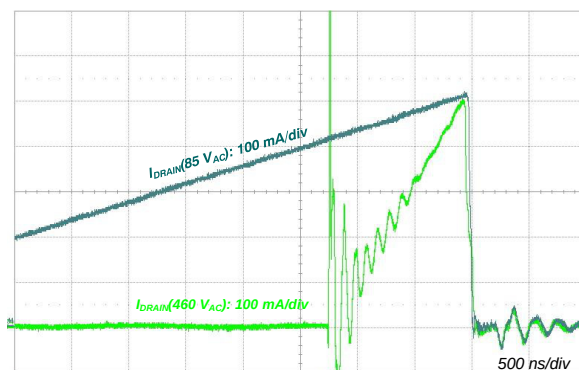
图 30. I_{LIM} 波形 (85 V AC 与 460 V AC )
