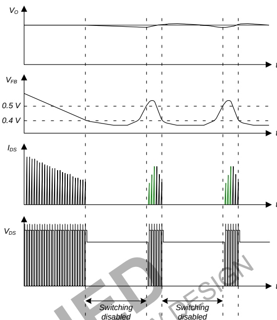
图 29. 间歇模式工作
