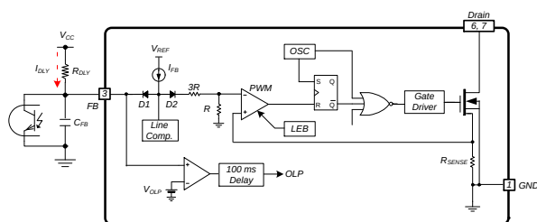
图 21. OLP 电路
