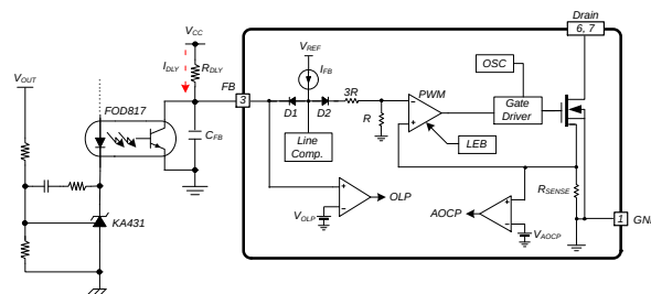
图 18. 脉宽调制电路
