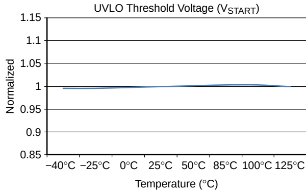
图 11. UVLO 阈值电压 ( V_{\text{START}} ) 与 T_A
