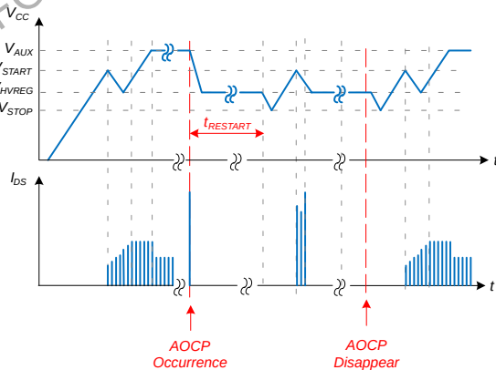
图 22. AOCP 波形
