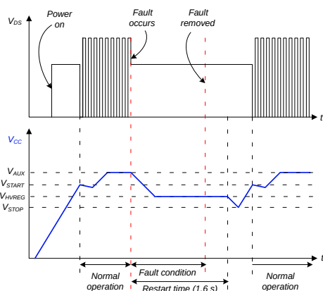
图 19. 自动重启保护波形
