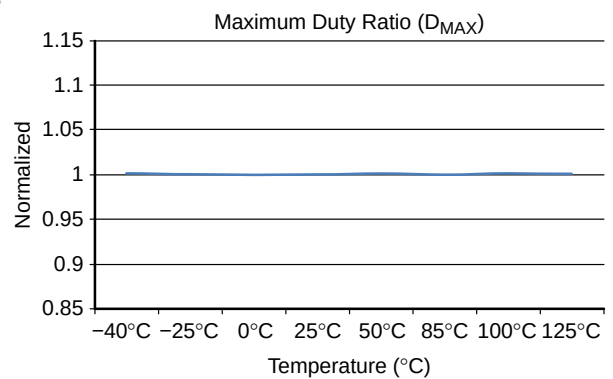
图 16. 最大占空比 ( D_{\text{MAX}} ) 与 T_A
