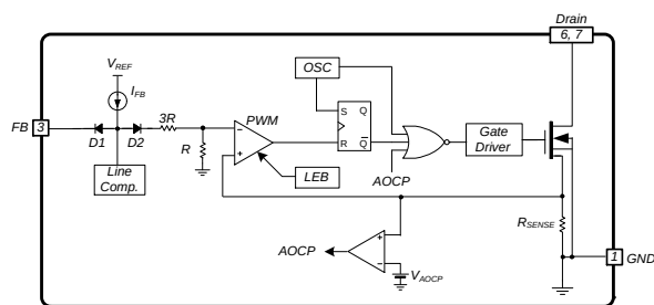
图 23. AOCp 电路
