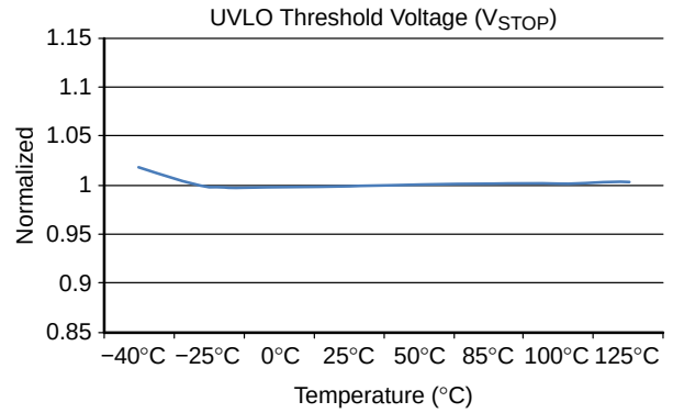
图 12. UVLO 阈值电压 ( V_{\text{STOP}} ) 与 T_A
