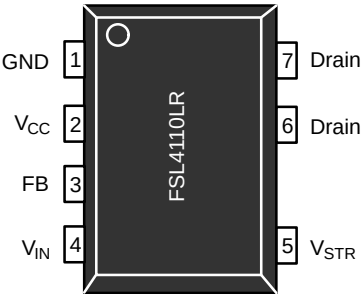
图 3. 引脚配置 (俯视图)
