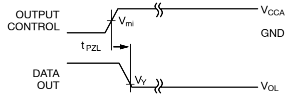
图 10. 3态输出低电平使能时间 (说明 18)
