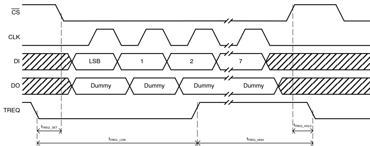
图 11. TREQ 时序图
