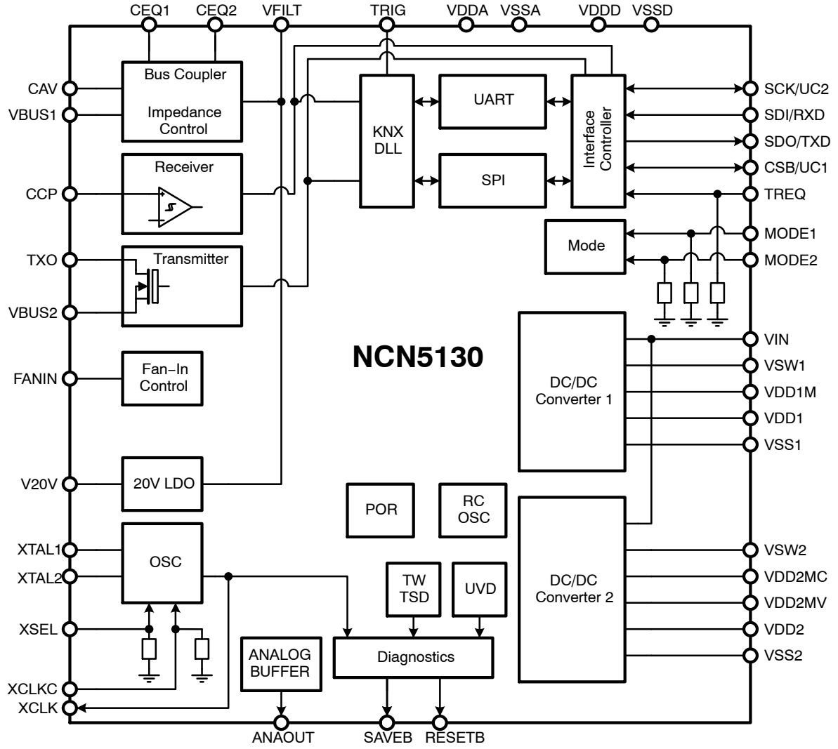
图 1. 框图 NCN5130
