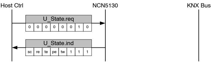
图 32. 状态服务
