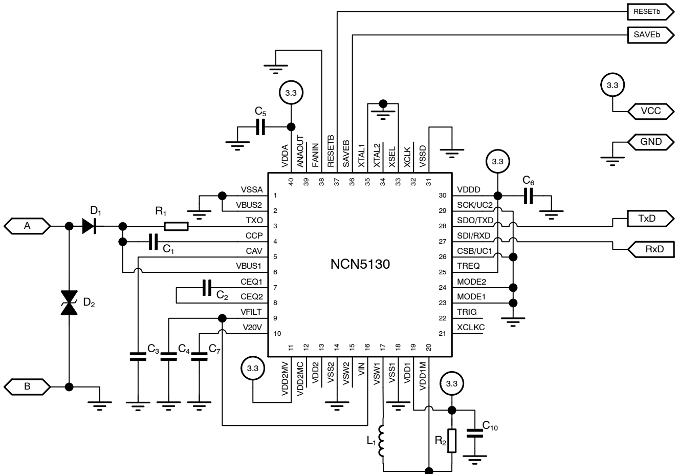
图 14. 典型应用原理图，模拟模式，单电源，20 mA 总线限流和 1.0 mA/ms 总线电流斜率
