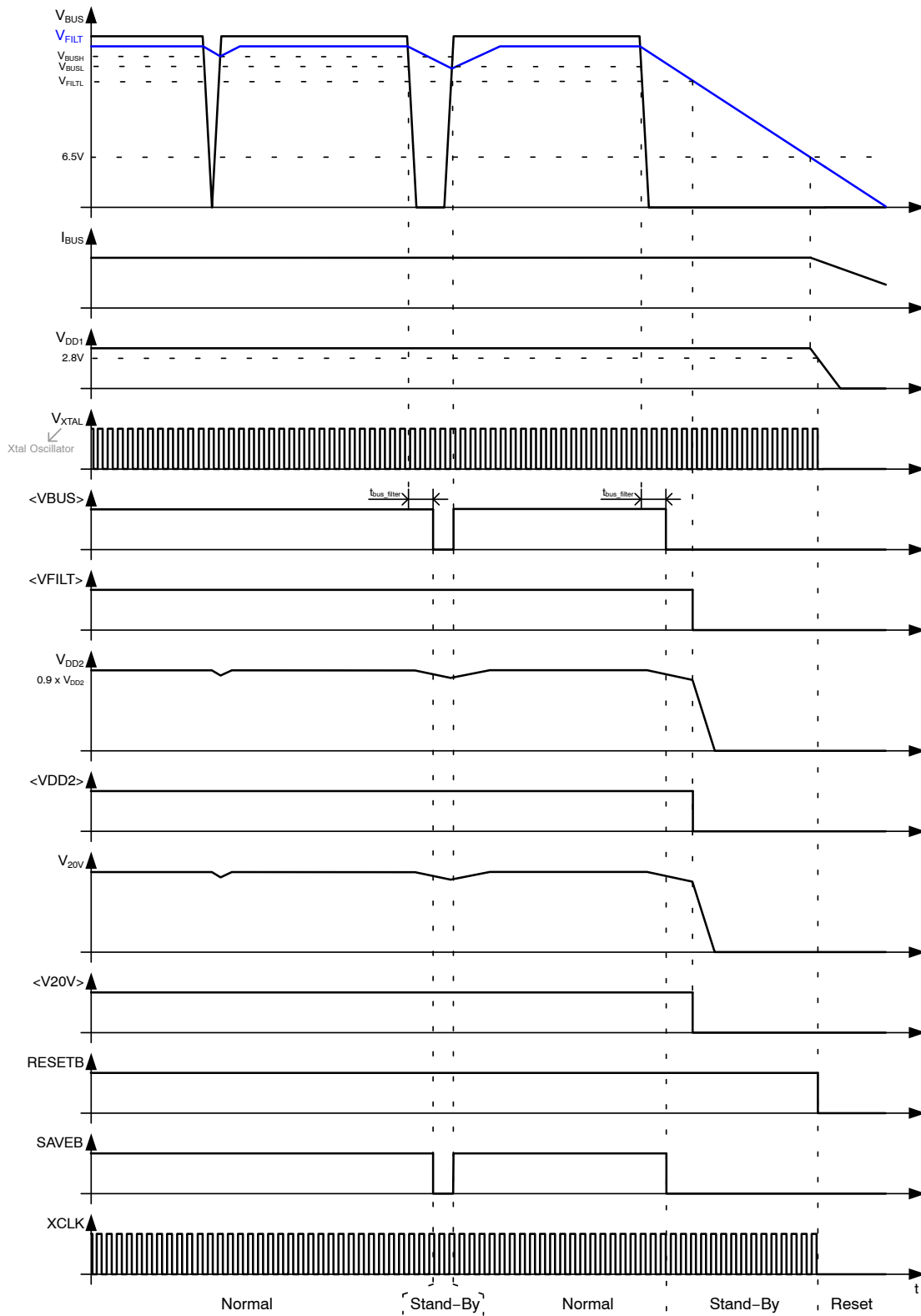
图 21. 关断行为
