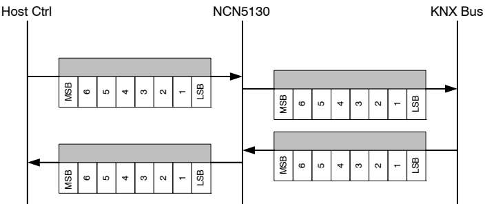
图 30. 服务的位序
