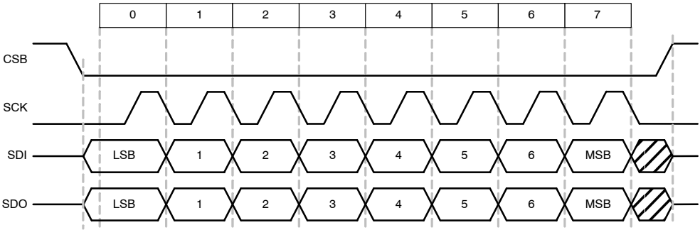
图 25. SPI 传输
