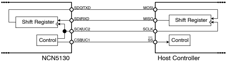
图 26. SPI 主机
