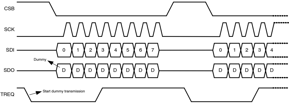
图 27. 传输请求
