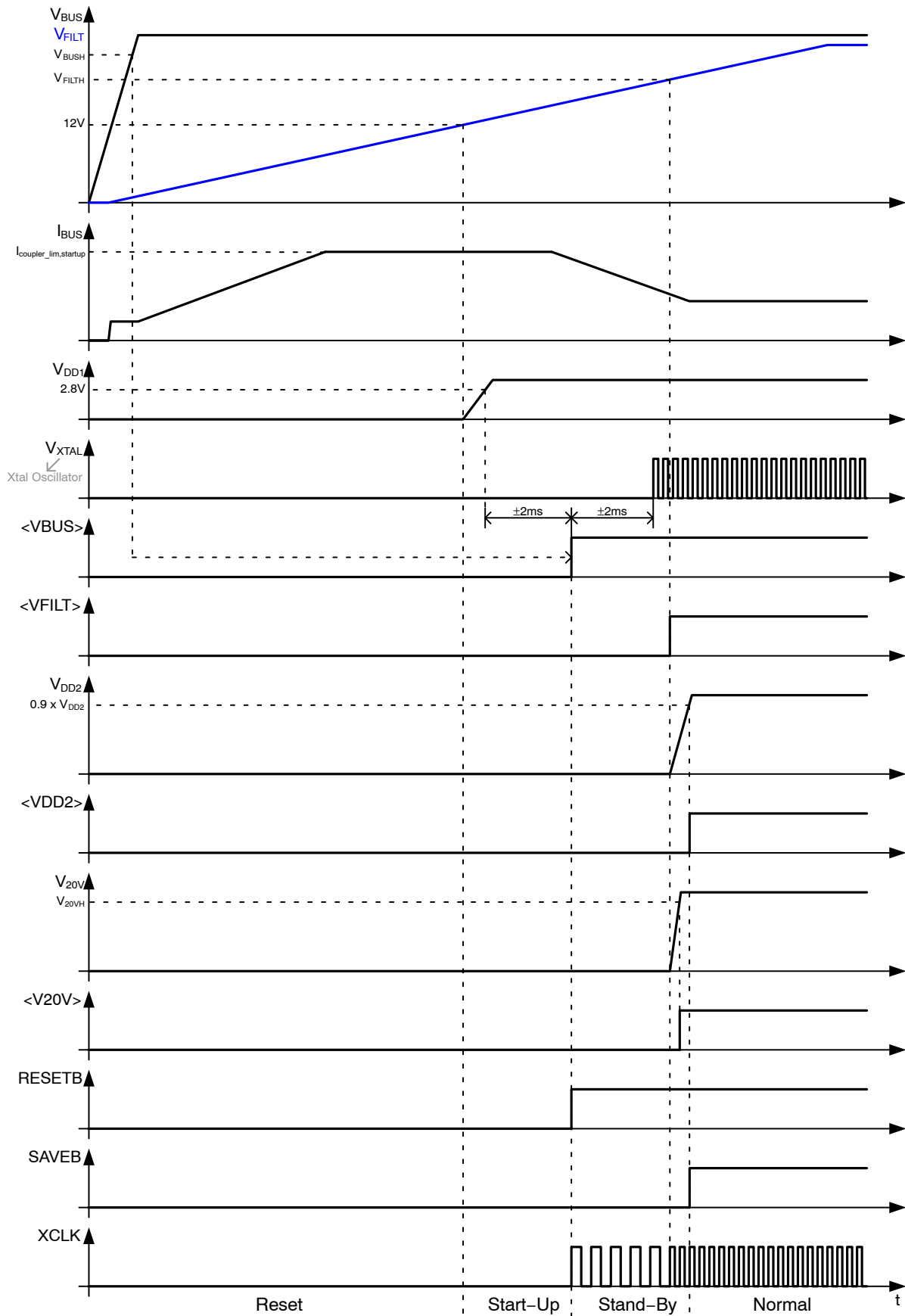
图 20. 启动行为
