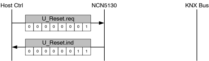
图 31. 重置服务
