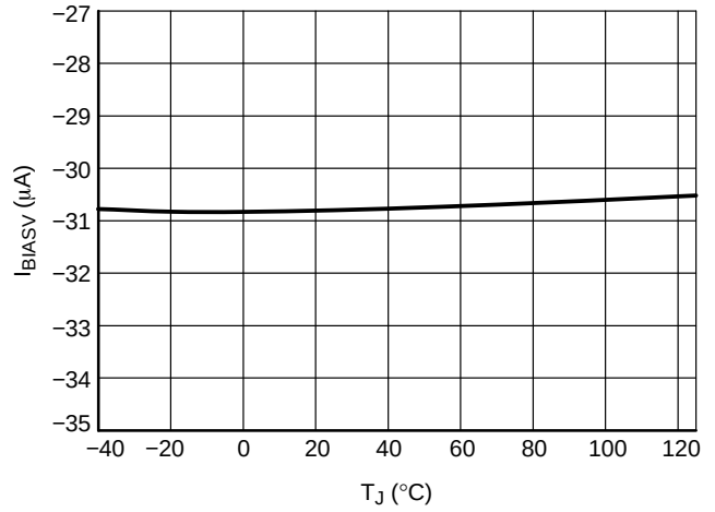
Figure 9. I_{BIASV} at V_{CC} = 15\text{ V} , V_{SNS} > V_{SNSBIASV} , V_{ECOTETH} < 10\% V_{CC}
