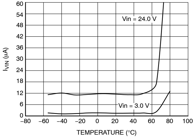
Figure 11. Vin Controller Current vs. Temperature (EN = 0)
