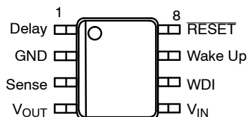
SOIC-8 EP
