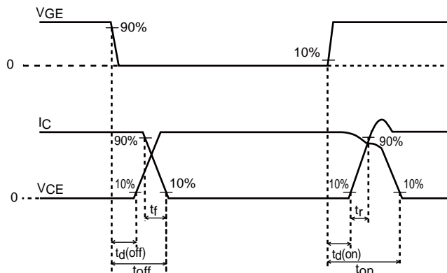
图 2 : 时间图
