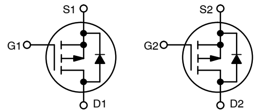
P-CHANNEL MOSFET
