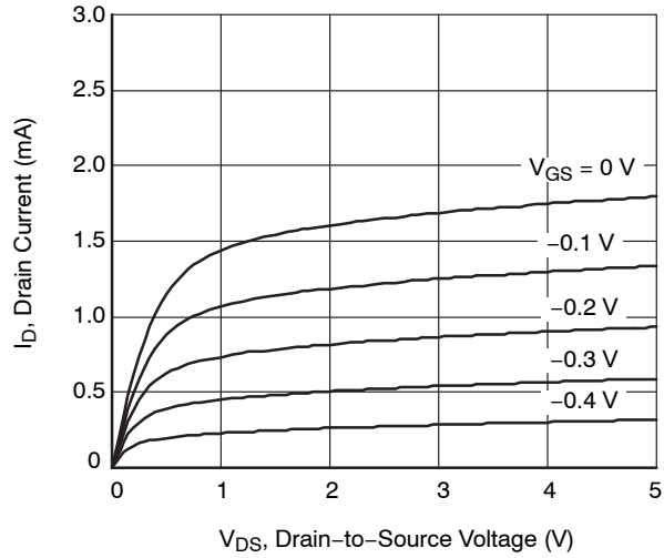
Figure 1. I_D - V_{DS}
