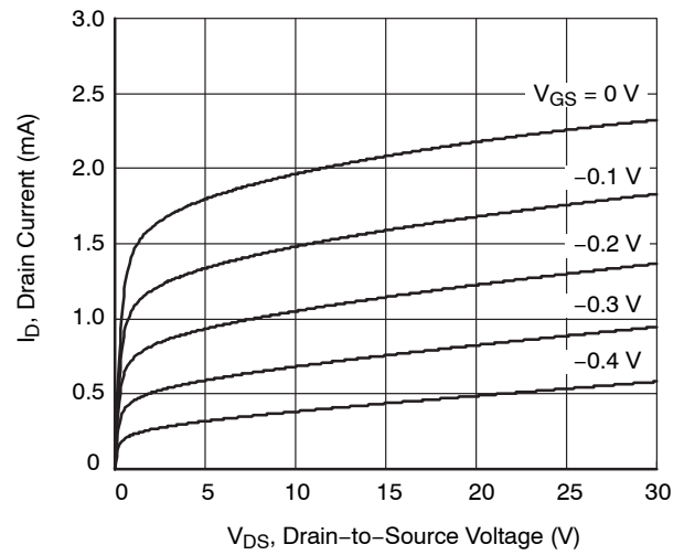
Figure 2. I_D - V_{DS}
