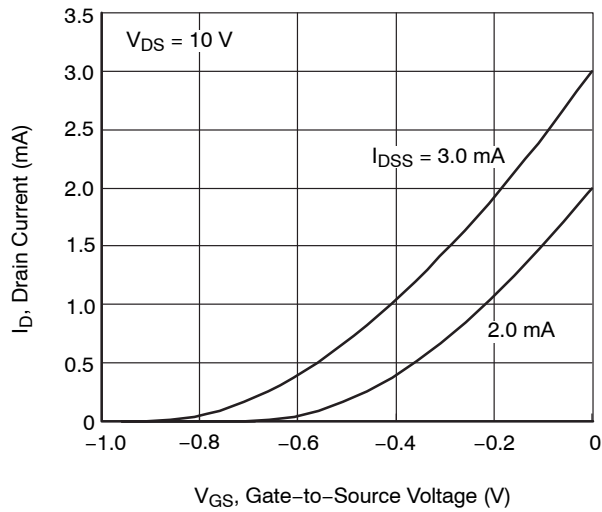
Figure 3. I_D - V_{GS}
