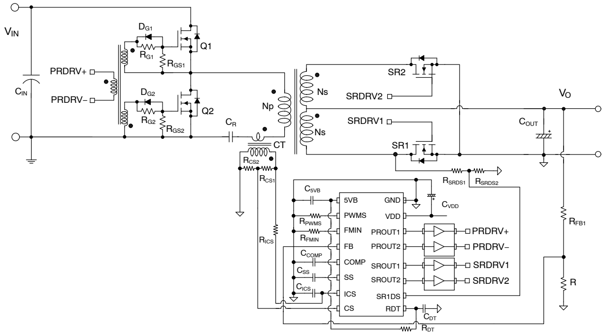
图 2. 典型应用
