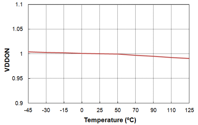
图 17. VDDON 与温度的关系
