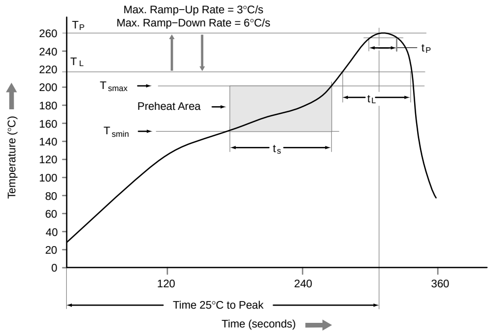
图 59. 回流焊数据
