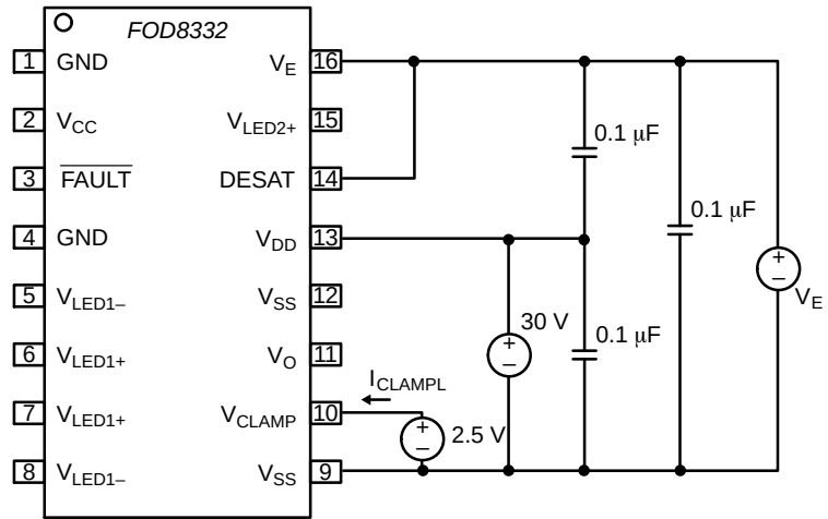
图 42. 箝位低电平灌电流 ( I_{\text{CLAMPL}} ) 测试电路
