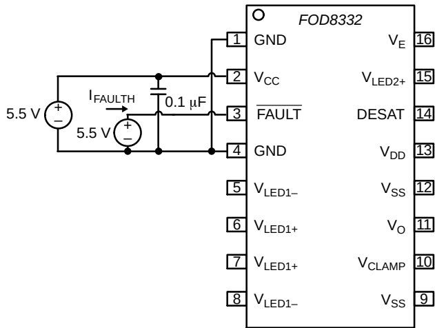
图 45. 故障高电平输出电流 ( I_{\text{FAULTH}} ) 测试电路
