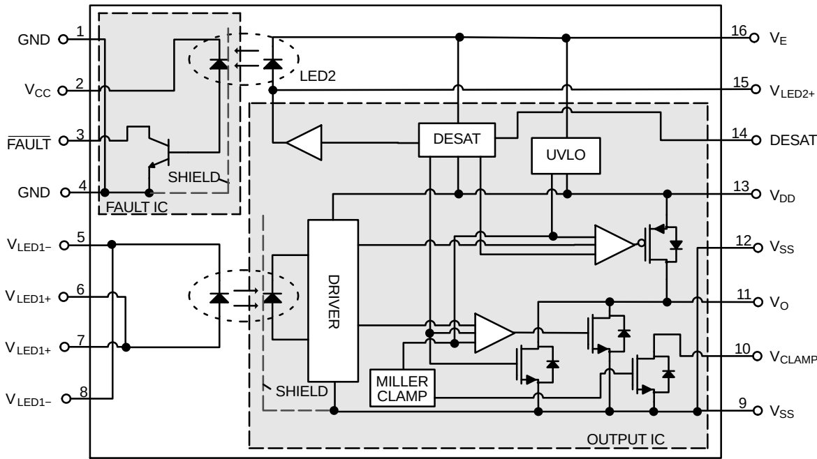
图 2. 功能框图
