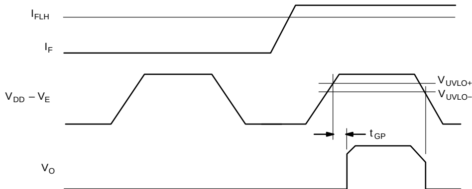
图 57. 供电时机
