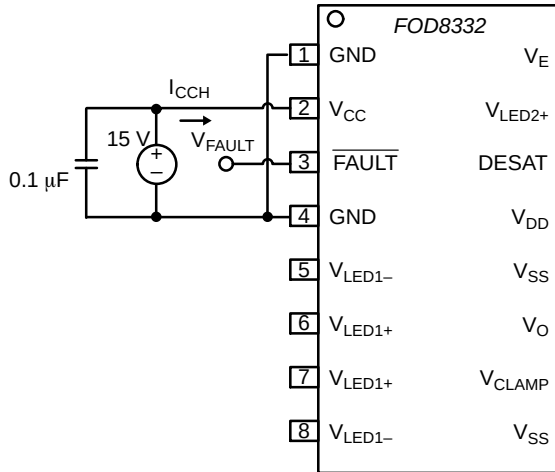
图 43. 故障高电平电源电流 ( I_{\text{CCH}} ) 测试电路
