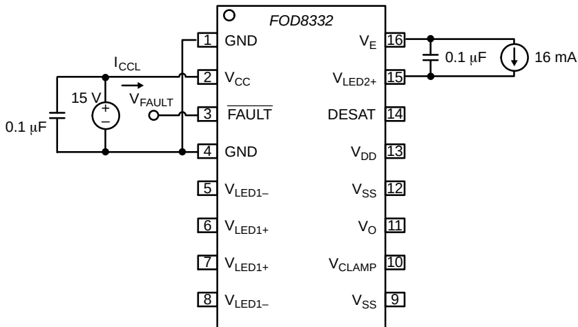
图 44. 故障低电平电源电流 ( I_{\text{CCL}} ) 测试电路
