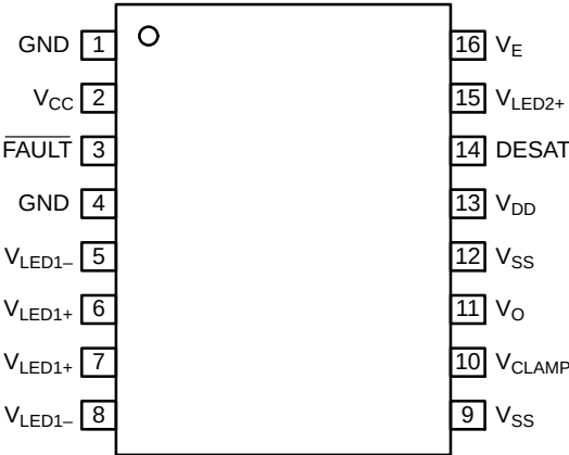
图 1. 引脚配置
