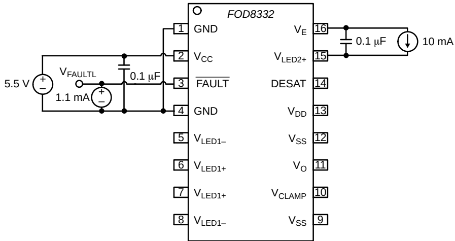
图 46. 故障低电平输出电压 ( V_{\text{FAULTL}} ) 测试电路
