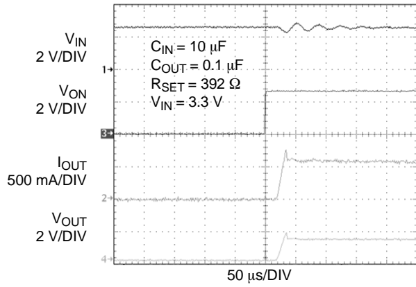
图 22. 电流限制响应时间 (输出的负载 2.2 \Omega , C_{OUT} = 0.1 \mu F )
