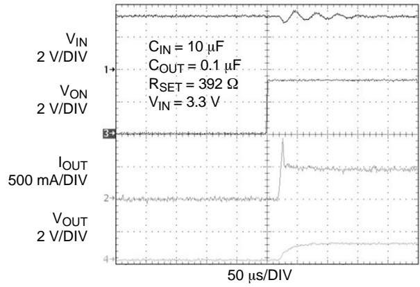
图 23. 电流限制响应时间 (输出的负载 2.2 \Omega , C_{OUT} = 10 \mu F )
