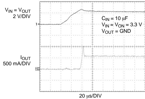
图 21. 电流限制响应时间 (开关短路)
