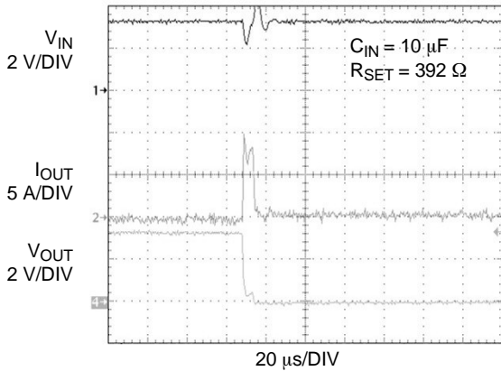
图 20. 短路响应时间 (输出短接至GND)
