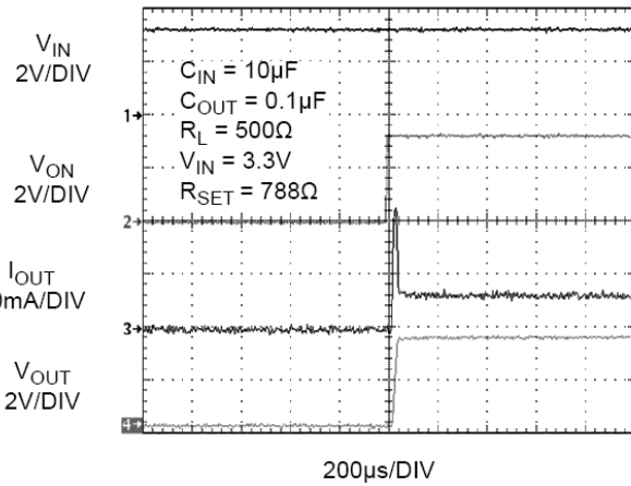
图18. t ON 响应
