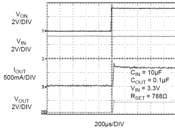
图22. 电流限制响应时间 (输出Ω C OUT = 0.1 µF)
