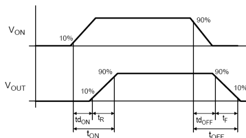
图27. 时序图
