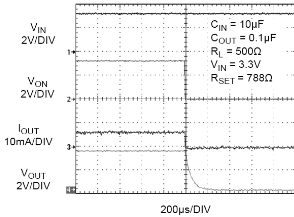
图19. t OFF 响应
