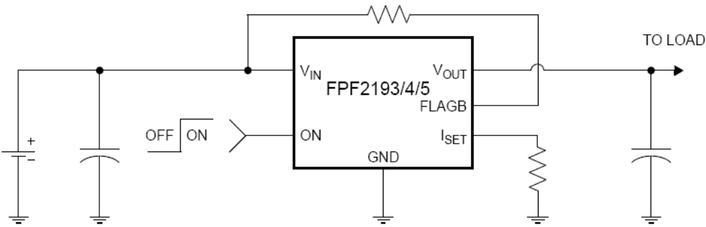
图1. 典型应用
