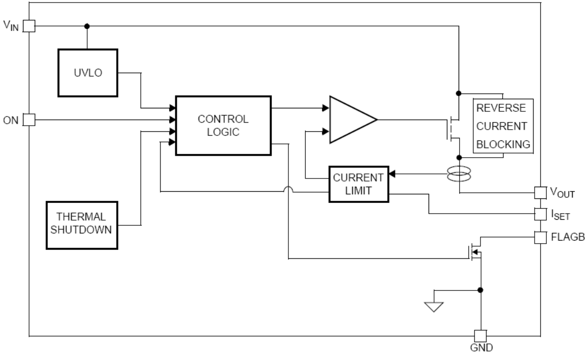
图2. 功能框图
