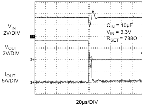
图20. 短路响应时间 (输出短路至GND)
