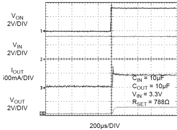
图23. 电流限制响应时间 (输出端 C_{OUT} = 10 \mu\text{F} )
