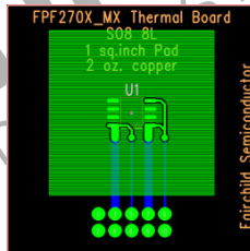
图 7. 102^\circ\text{C/W} , 安装在一个 2-oz 的 1\text{in}^2 焊盘上铜
