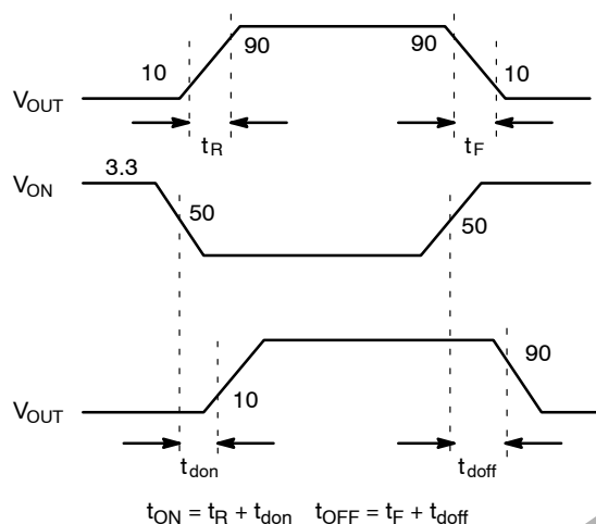
图 9. 时序图
