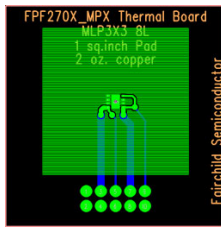
图 5. 80^\circ\text{C/W} , 安装在一个 2-oz 的 1\text{in}^2 焊盘上铜
