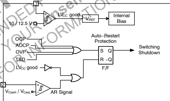
图 22. 保护框图
