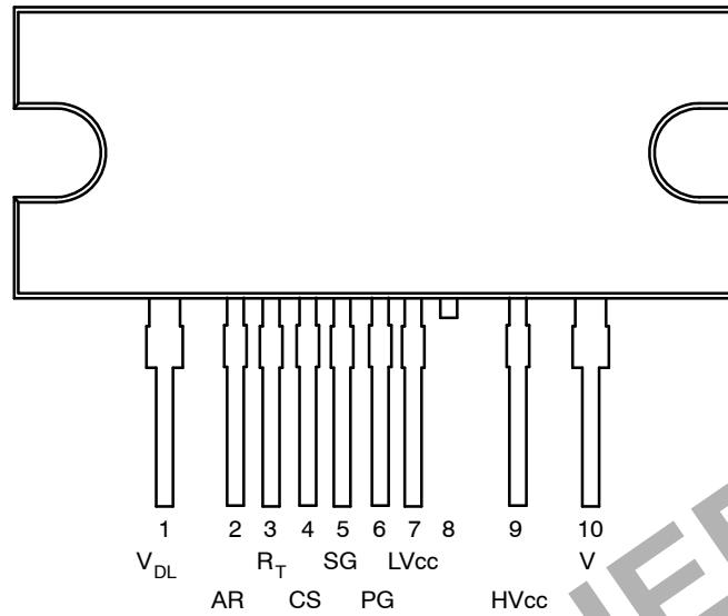
图 3. 封装图
