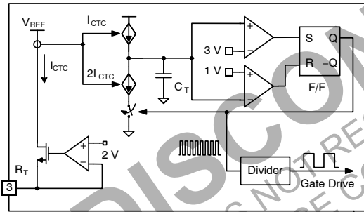
图 16. 电流控制的振荡器
