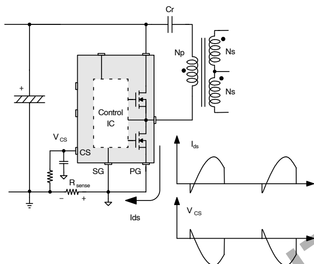
图 23. 半波检测
